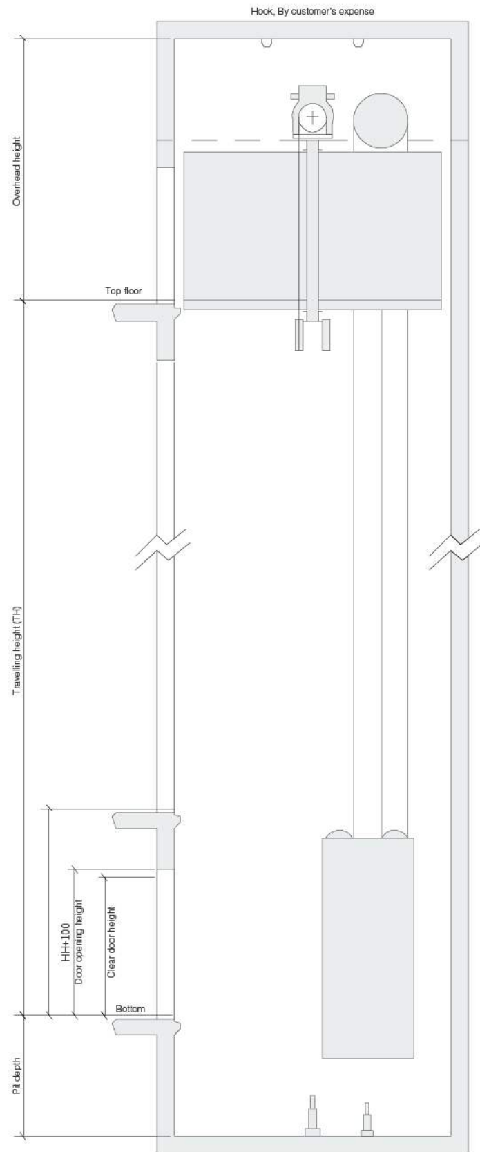
Hoistway Elevation
