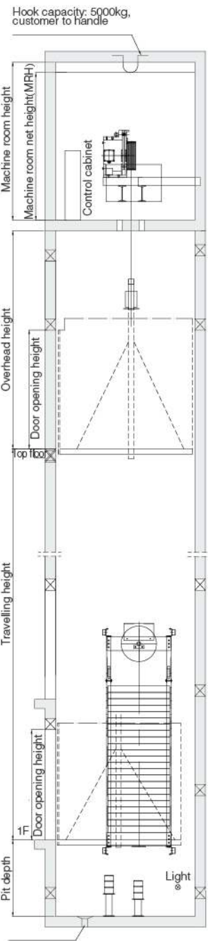
Hoistway Elevation
