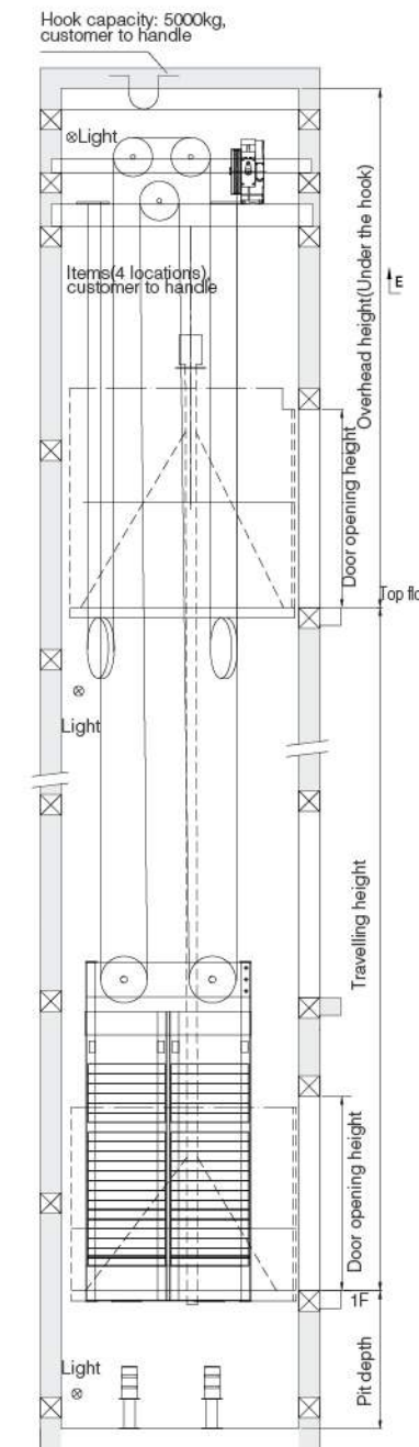
Hoistway Elevation
